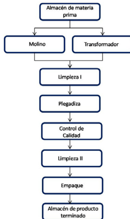
Diagrama de flujo del proceso de trabajo. Área de producción, Empresa papelera, México, 2012
